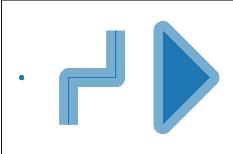
s.buffer(0.2, cap_style=2)
