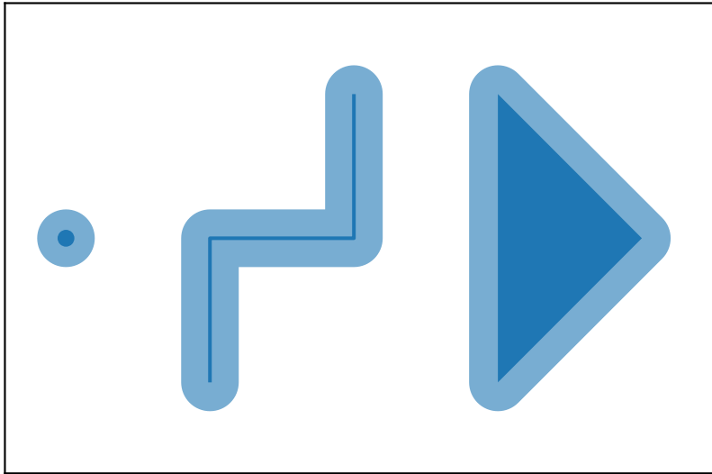
s.buffer(0.2)
