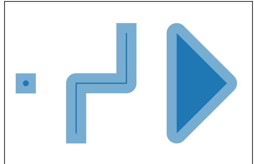
s.buffer(0.2, cap_style=3)
