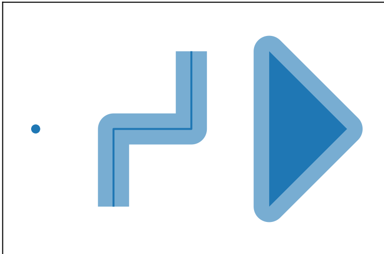
s.buffer(0.2, cap_style=2)
